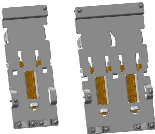
适用于 FSAA/FSAB/FSAC/FSA 的 DIN 导轨安装套件
